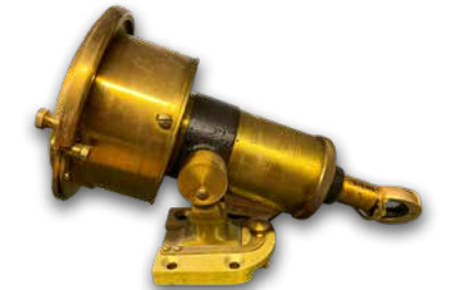
Reloj indicador de corredera de patente para medir la velocidad en millas, por Thomas Walker & Son, siglo XX. MNF-724
