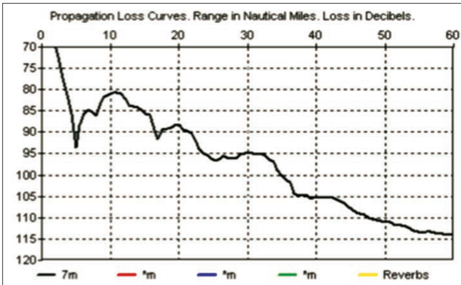
Gráfico 2.—Curva PROPLOS mar de Alborán, mes de octubre, obtenida por el programa WADER 32.
