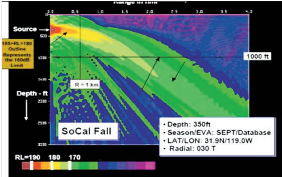
Niveles de exposición sonora de propagación del sonar LFA-SURTASS.
