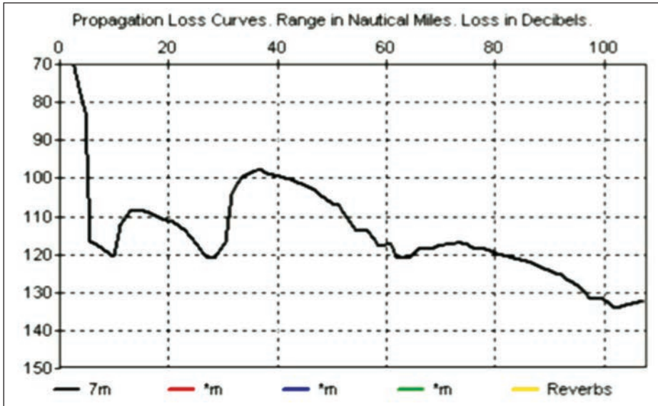
Gráfico 1.—Curva PROPLOS océano Atlántico, mes de febrero, obtenida por el programa WADER 32.
