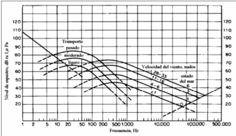
Espectros medios del ruido ambiental de las aguas profundas. ( http://mit.ocw.universia.net/13.00/NR/rdonlyres/D629E305-6EC8-4664-B7A4-AF44152E54B4/0/1300_acoustics_lecture_notes.pdf ).
