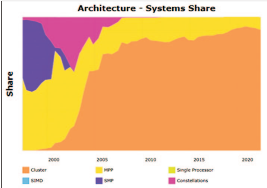
Ilustración 2. Arquitecturas empleadas en los supercomputadores del TOP500 entre los años 1997 y 2022
