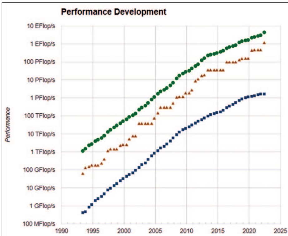
Ilustración 1. Capacidad de cómputo de los supercomputadores del TOP 500
